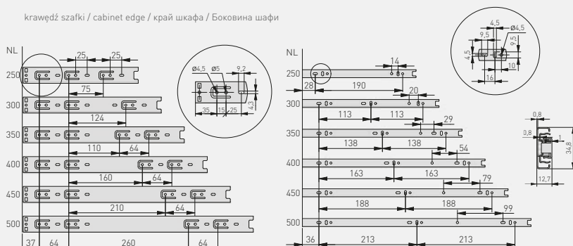
krawędź szafki / cabinet edge / край шкафа / Боковина шафи
