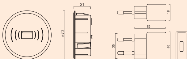
Wymiary ładowarki
